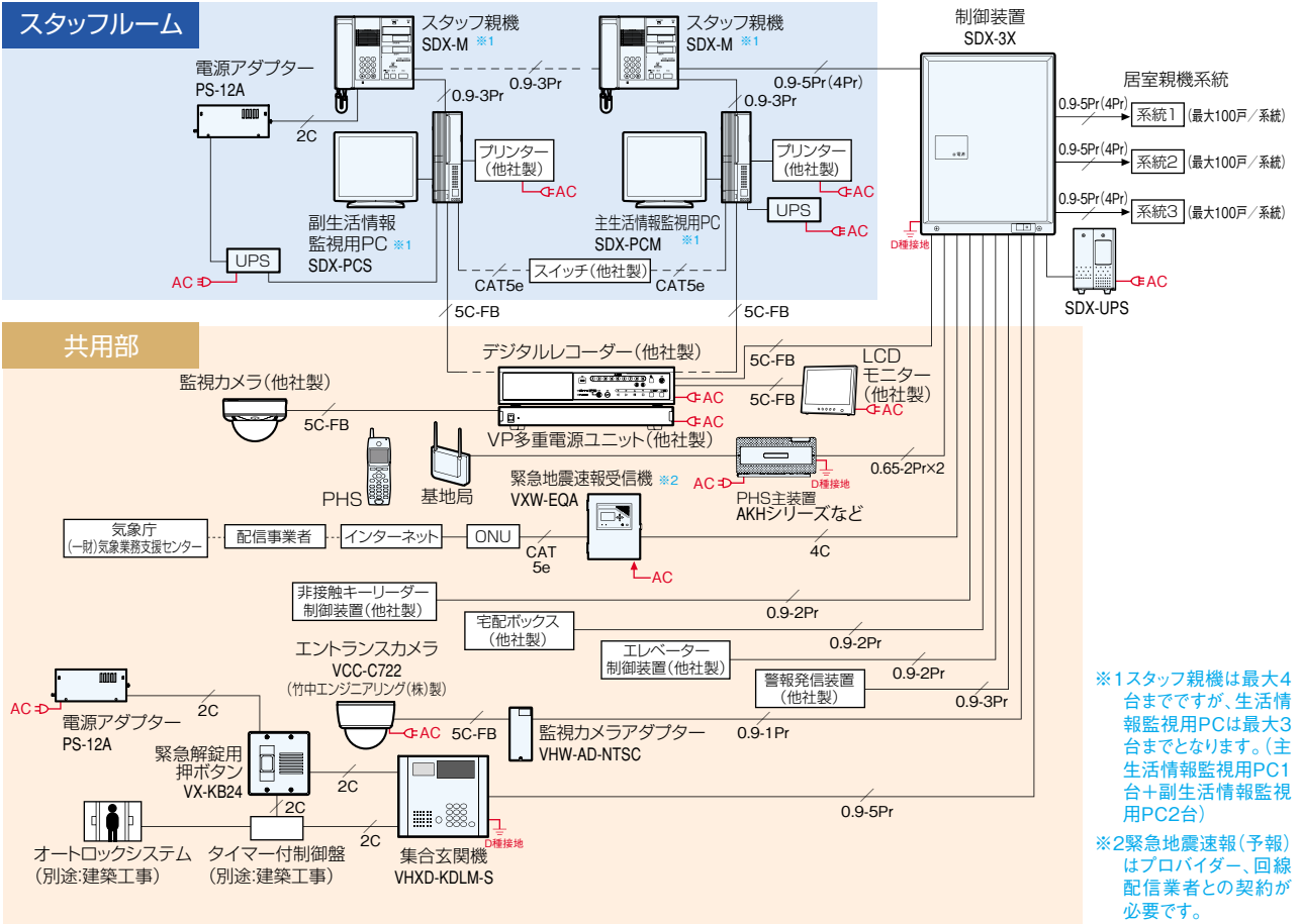
FAGUS (2通話路・2映像路システム例)
