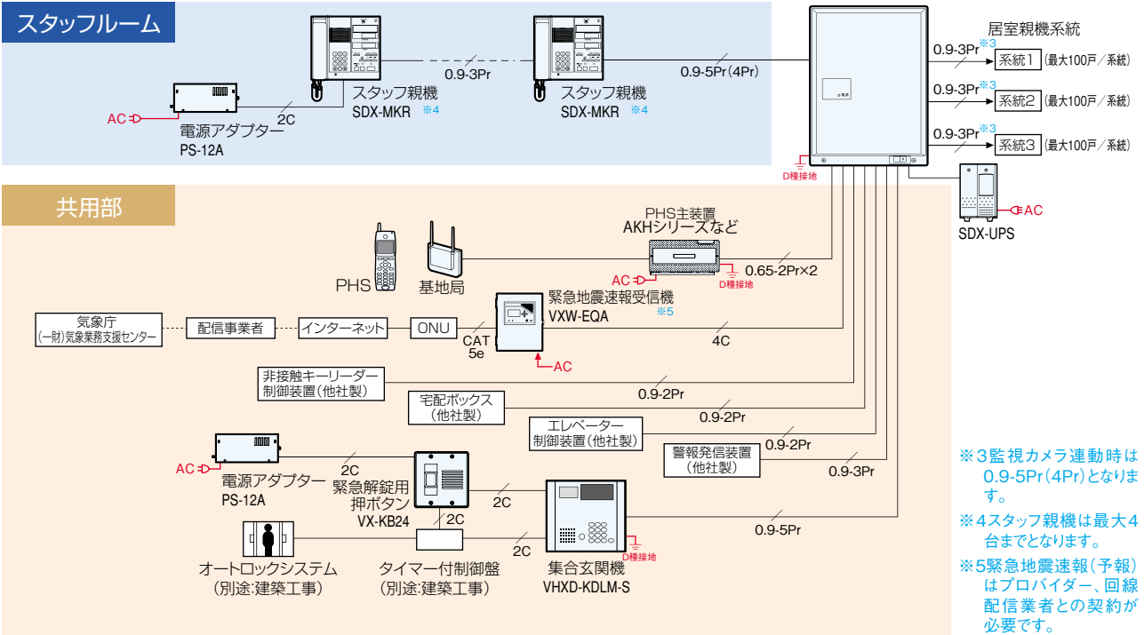
FAGUS ライト (2通話路・2映像路システム例)
