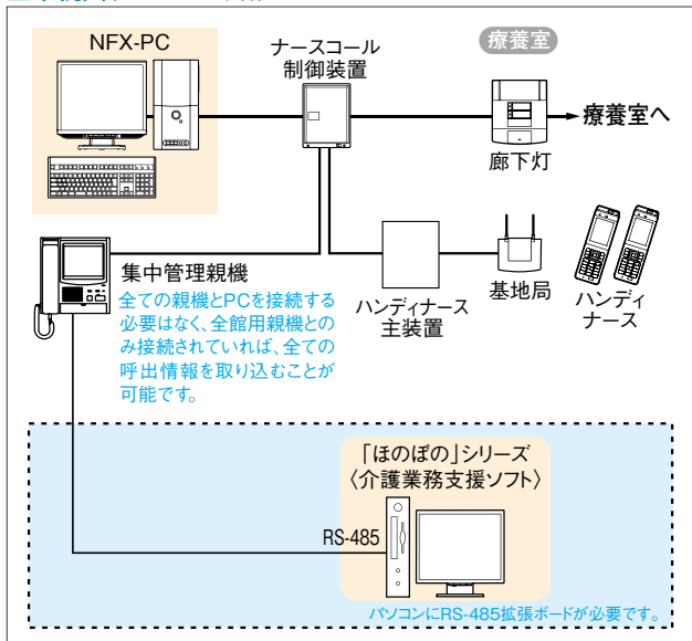
■系統図 (NFX-PCの場合)
