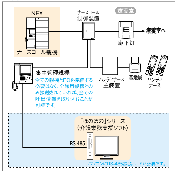
■系統図 (NFXの場合)
