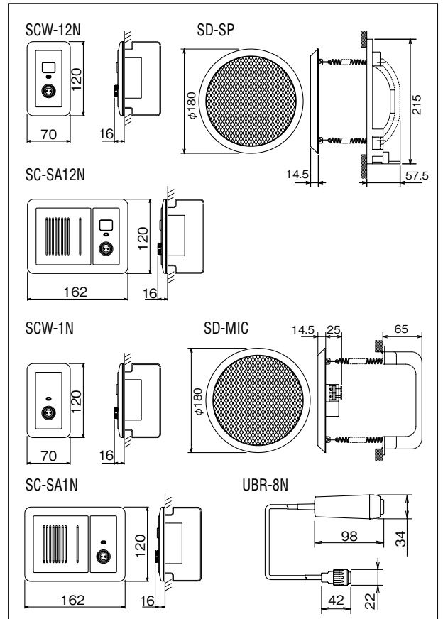
天井埋込型マイク SD-MIC 市販品 希望小売価格 4,600円(税別) ●埋込型
