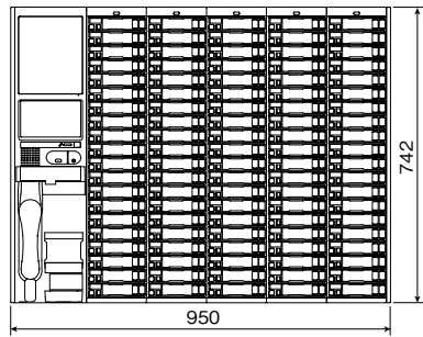
NLX-MBUC+NLX-20BU×5台 (100局)
