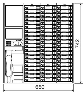
NLX-MBUC+NLX-20BU×3台 (60局)
