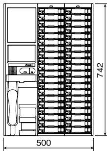
NLX-MBUC+NLX-20BU×2台 (40局)
