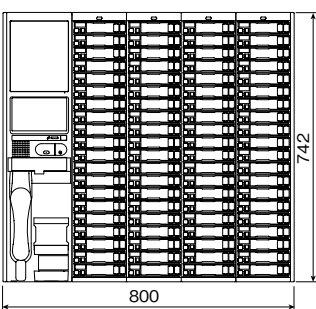
NLX-MBUC+NLX-20BU×4台 (80局)
