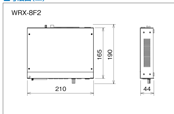
■寸法図(mm)
