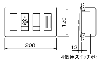
4個用スイッチボックス
