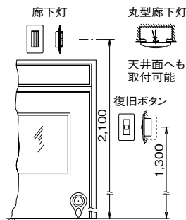
1個用スイッチボックス
