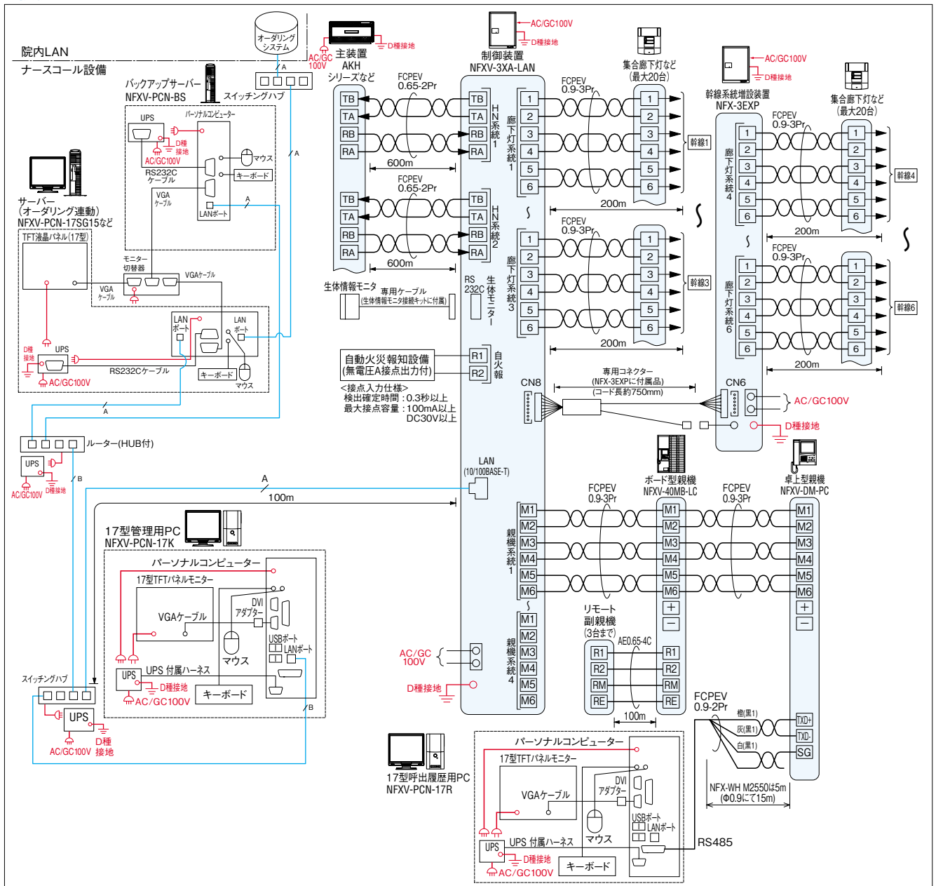
■ 接続図
