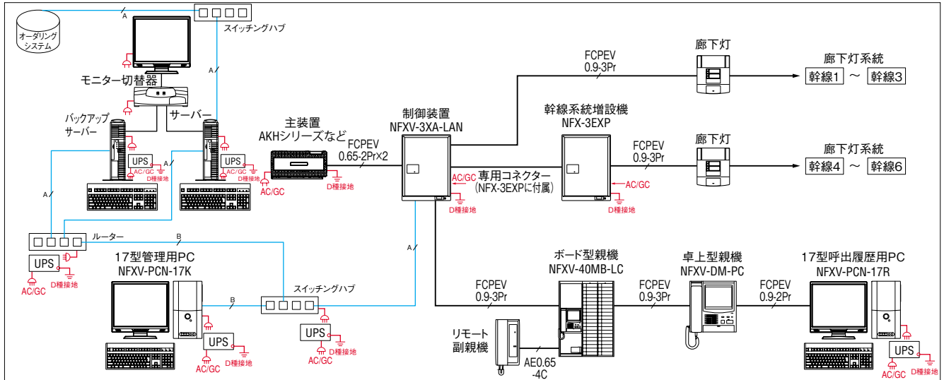
■ 系統図
