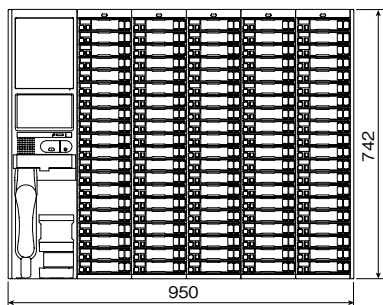
NLX-MBU+NLX-20BU×5台 (100局)
