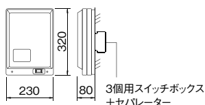
VHXW-1X-1
