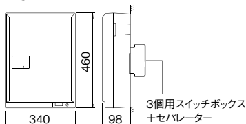
VHXW-3X(W)-2、VHXW-6XW-2、RVHXW-6XW-1、RVHXW-3XW-1
