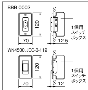
非常ボタン(プレート別) JEC-B-119(市販品) ※神保電器(株)製
