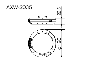
取付ベース トリツケベースA ¥700(税別) ※パナソニック(株)製
